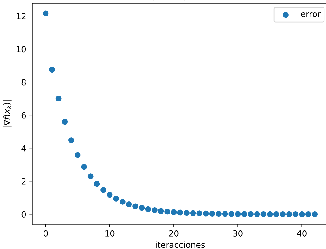
Gráfica |\nabla f(x_k)| de funcion i
